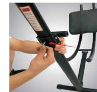
ПОДВИЖНОЕ УСТРОЙСТВО В ВЕРТИКАЛЬНОЙ НАПРАВЛЯЮЩЕЙ Совместите отверстие в втулке основной трубы с отверстием в вертикальной трубе, и закрепите их, используя штифт из комплекта поставки.
